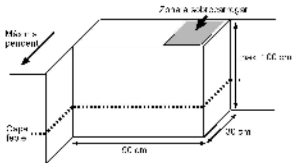
Figura 2: Diagrama de les mides del bloc a aïllar en l'ECT (modificat de Simenhois & Birkeland 2006) i fotografia d'un ECT positiu aquest hivern al Pirineu.
