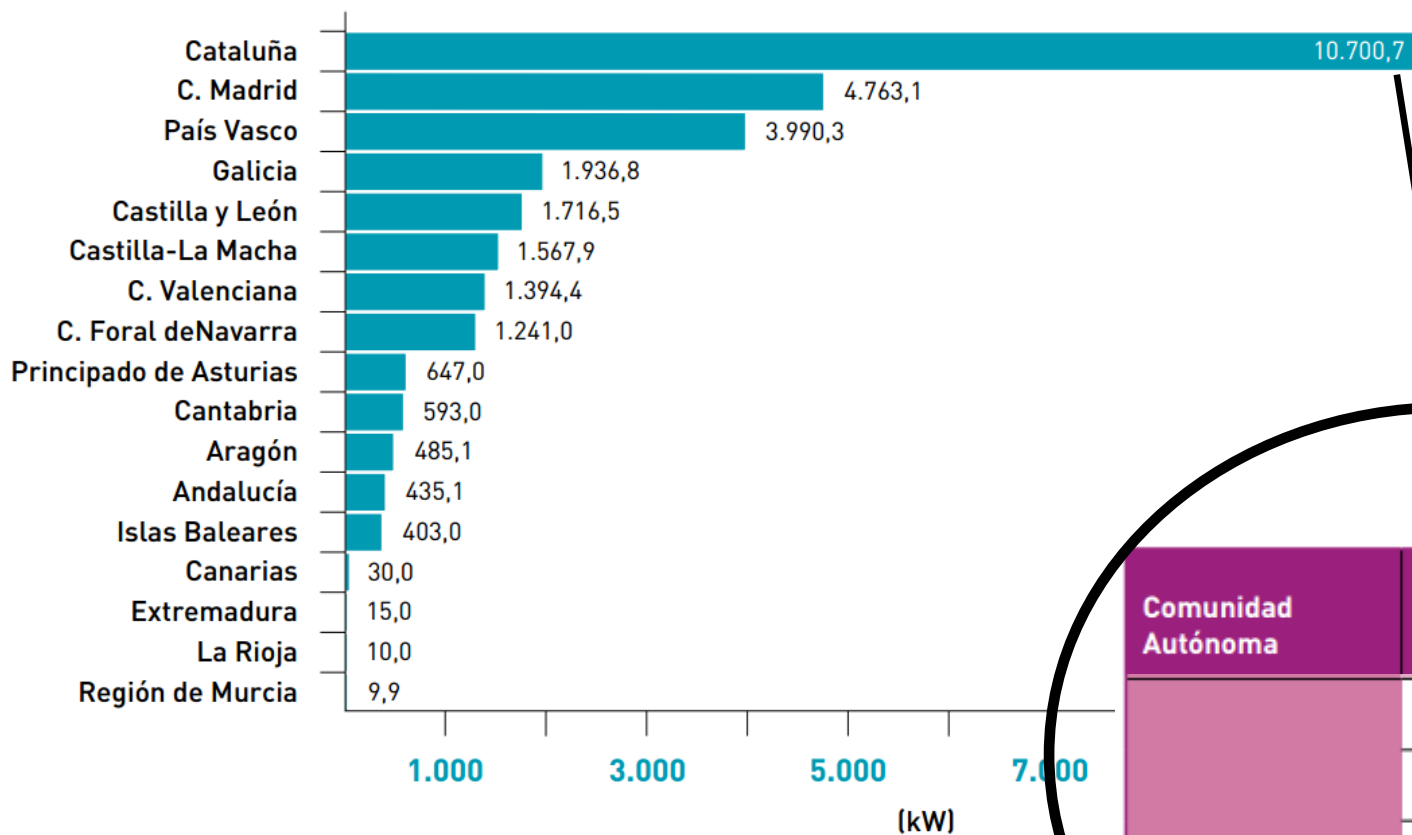
Figura 9.3. Distribución por CC AA de la potencia térmica instalada
